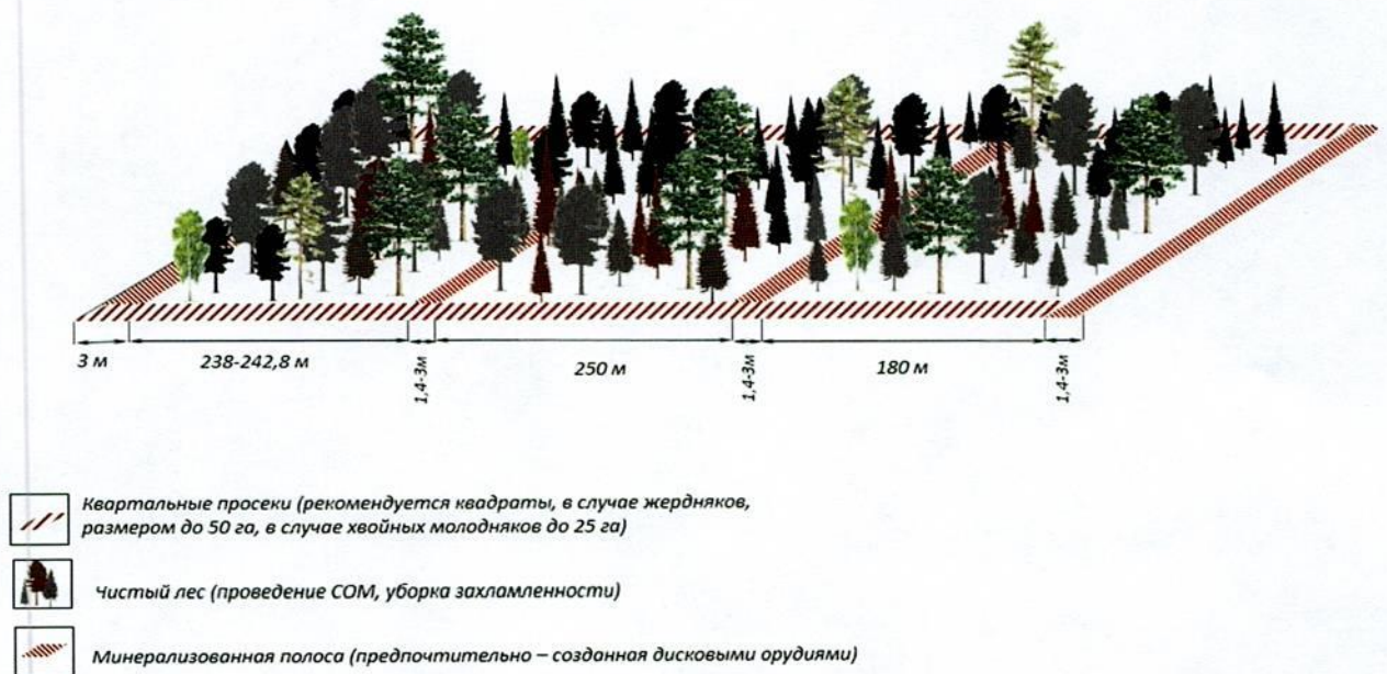
Типовая схема противопожарного обустройства насаждений, в которых вероятно развитие верховых пожаров (вторая подзона)
