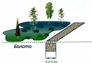
Противопожарная канава в разрезе (предлагаемый вариант)
