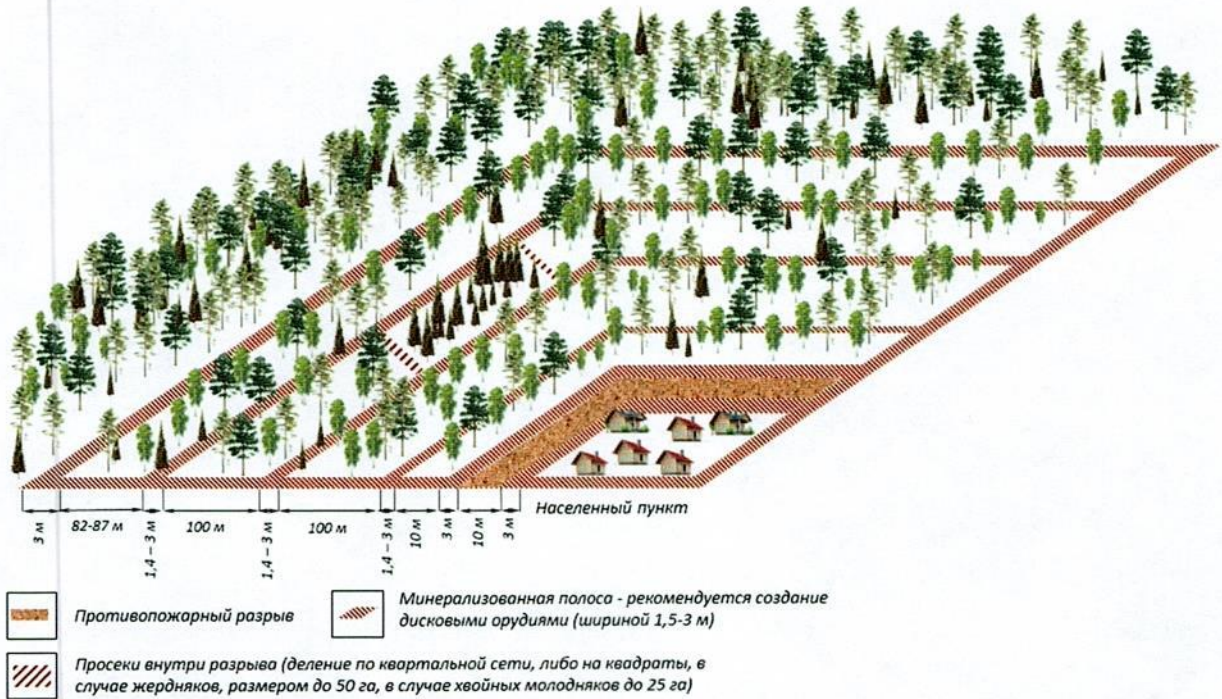
Типовая схема противопожарного обустройства насаждений, в которых вероятно развитие верховых пожаров (первая подзона)
