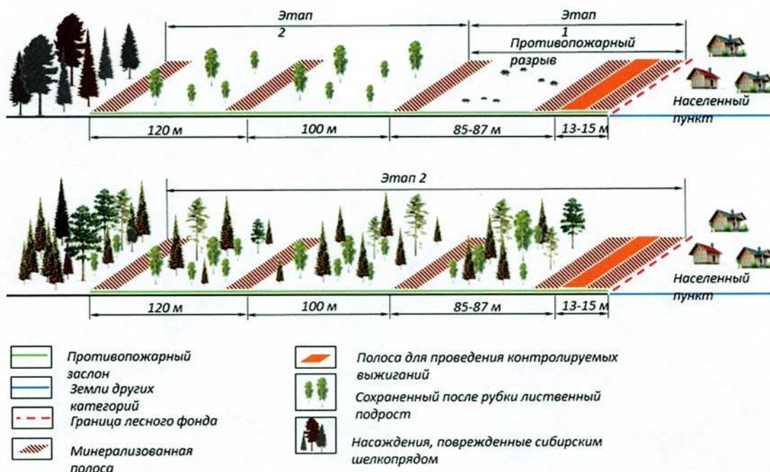
Типовая схема противопожарного обустройства первой зоны сильно захламленных нарушенных участков лесных земель
