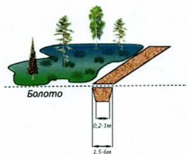
Противопожарная канава в разрезе (ГОСТ Р 57972-2017)
