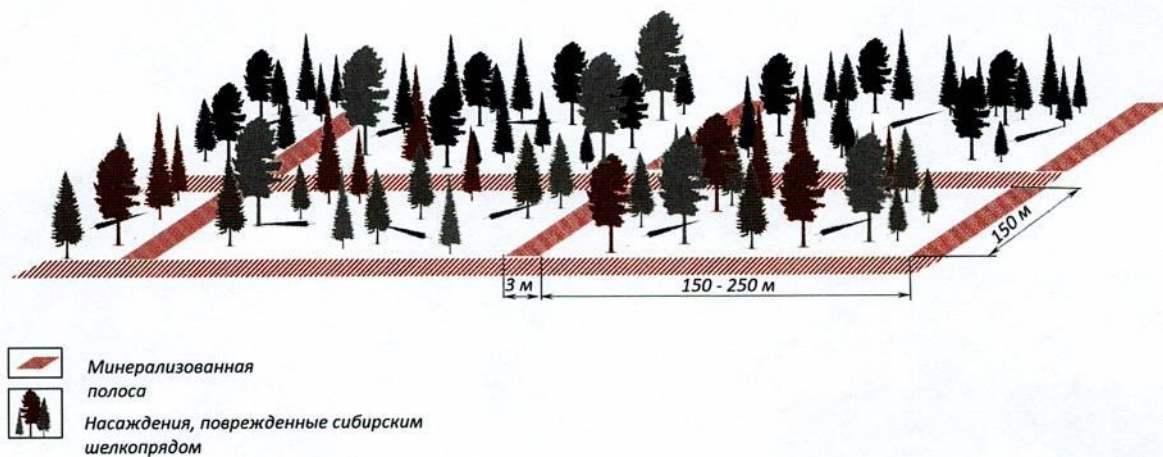
Типовая схема противопожарного обустройства сильно захламленных нарушенных участков лесных земель (вторая подзона)
